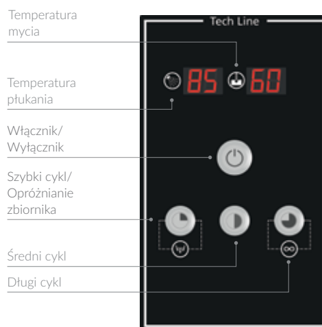
Panel sterujący
