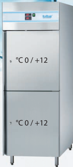
Szafa chłodnicza 2-temperaturowa GN 2/1 drzwi skrzydłowe ze stali szlachetnej z podwójnymi ściankami 2-temperature refrigerator GN 2/1 with 2 separately-adjustable refrigeration compartments for normal refrigeration
